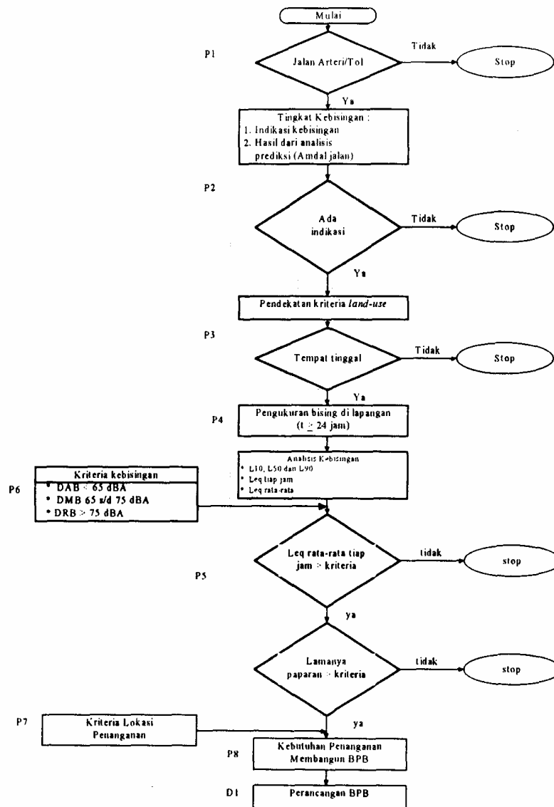
Gambar 1. Diagram Alir Proses Perencanaan dan Perancangan
