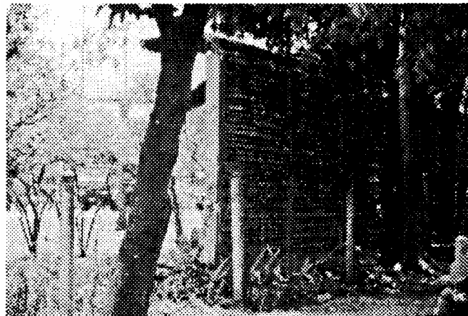
Gambar 2. Dinding Peredain Bising yang terbuat dari Bata Merah
