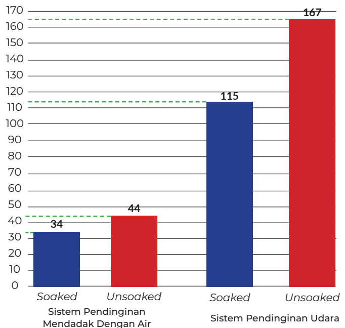
Gambar 3. Resume pengujian CBR untuk Limbah slag nikel
