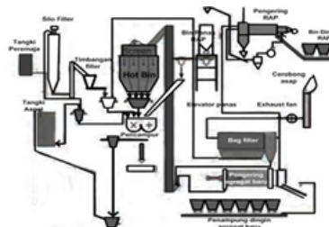
Gambar 4. Unit Pencampur Campuran Beraspal Panas Daur Ulang Sistem Timbangan Untuk RAP Panas (Nono, 2018)
