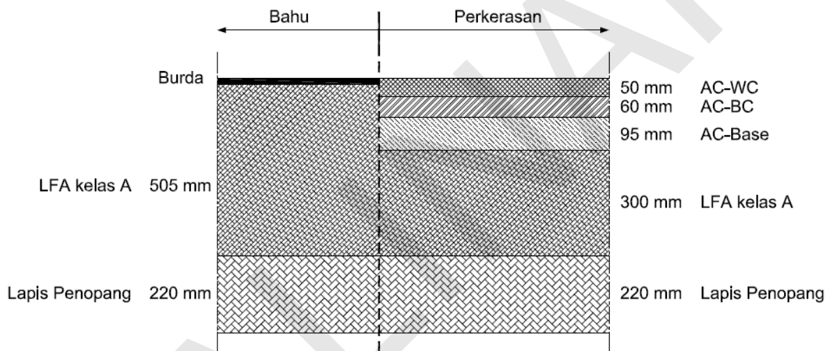
Gambar 10.8. Alternatif Struktur Perkerasan Bahu Jalan pada Grade > 4%
