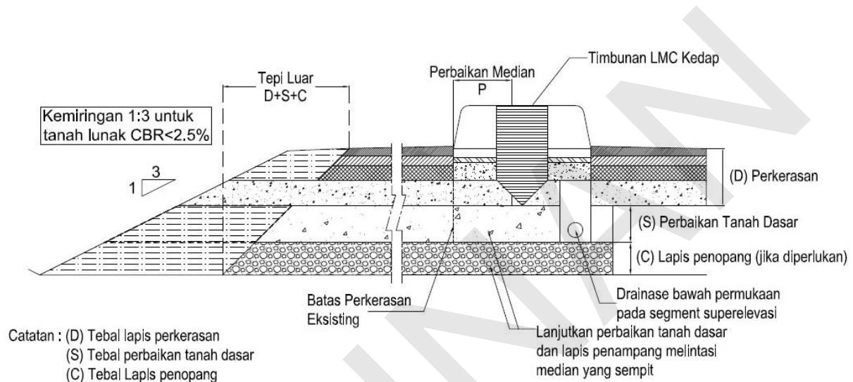
Gambar 8.1. Dukungan Tepi Perkerasan.
