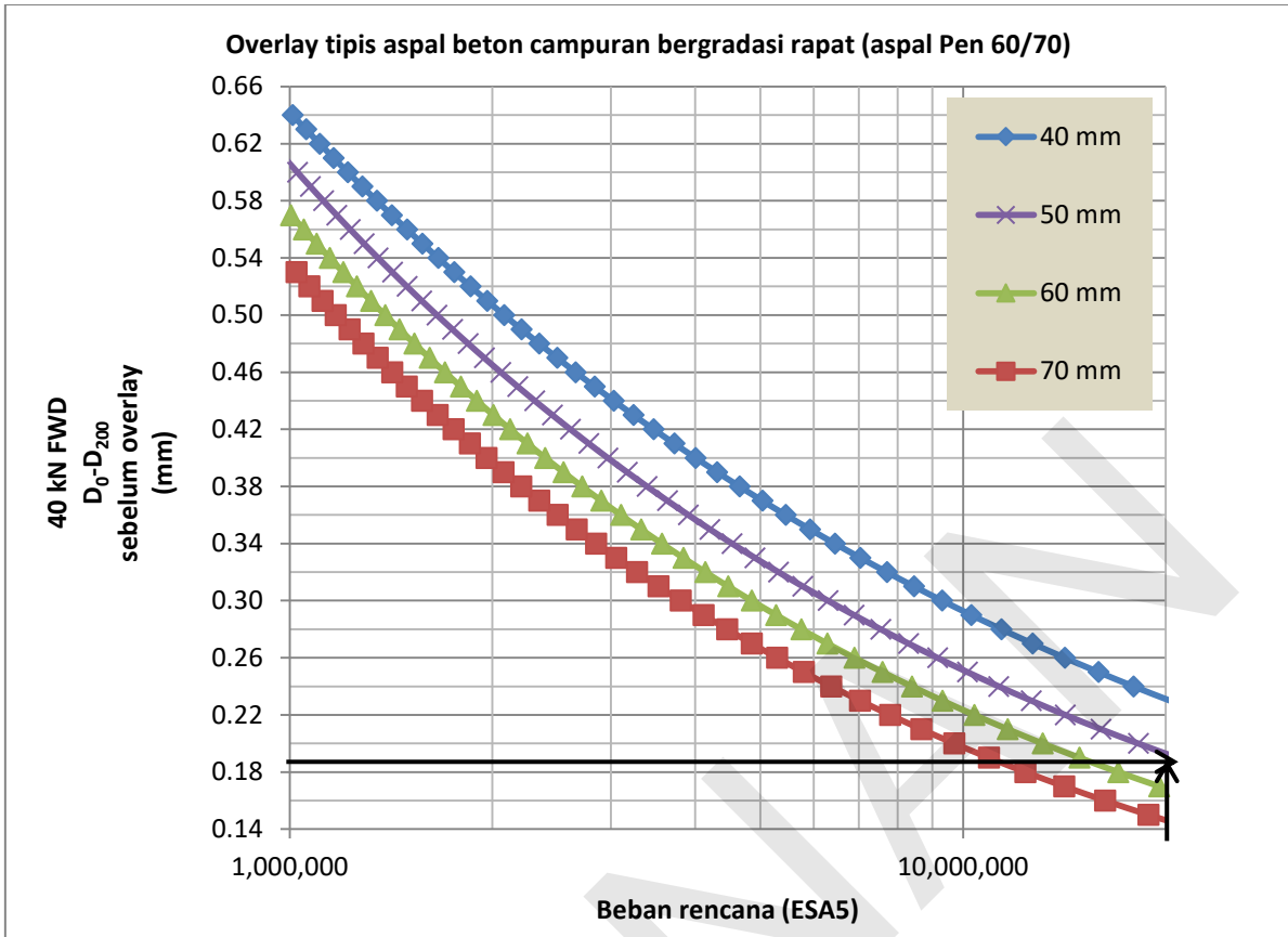
Gambar 10.2. Penetapan Tebal Overlay (tipis)
