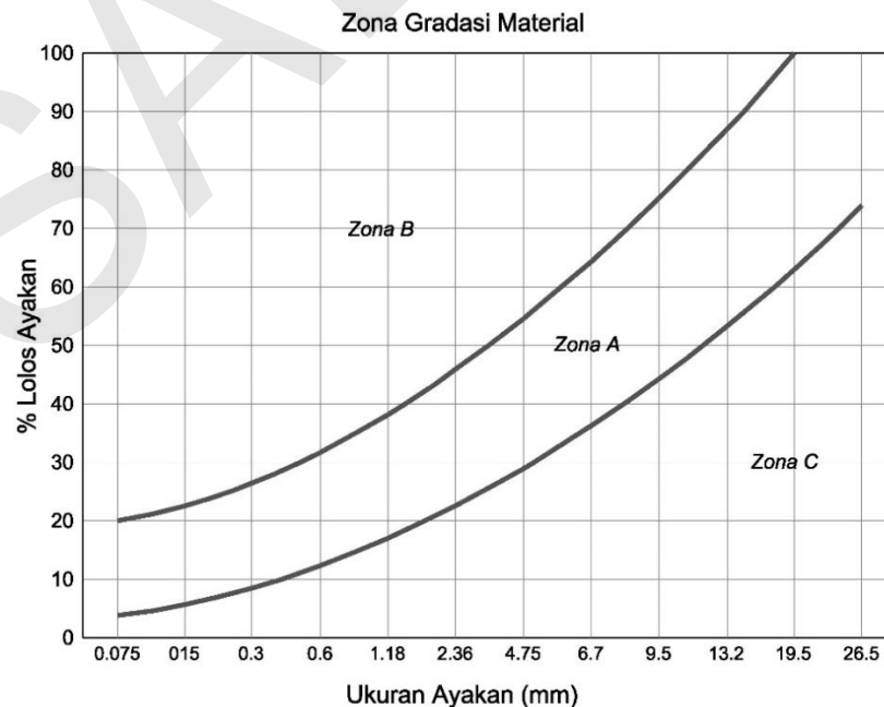
Gambar 8.2. Amplop Gradasi Zona A
