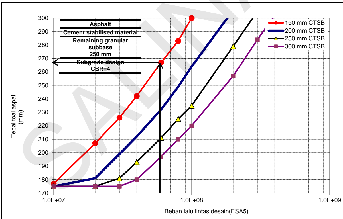
Gambar 10.5. Penentuan Tebal Lapisan CTSB dan Aspal
