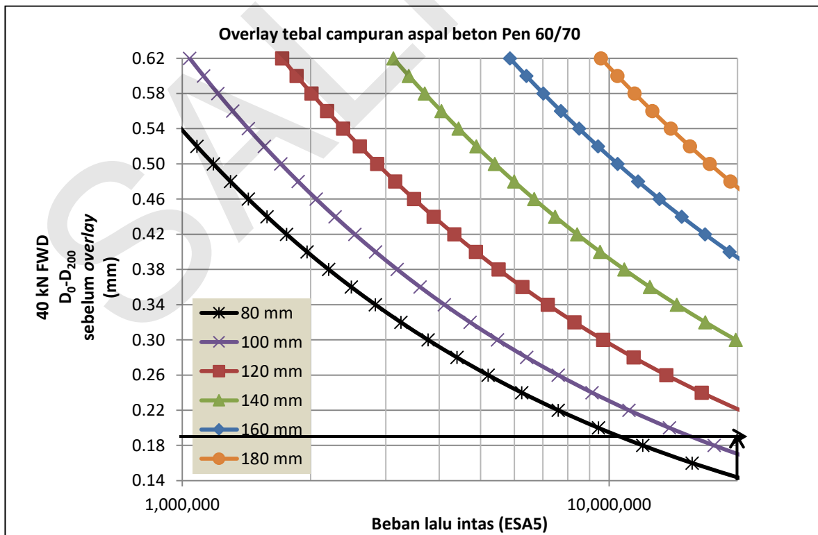
Gambar 10.3. Penetapan Tebal Overlay (tebal)
