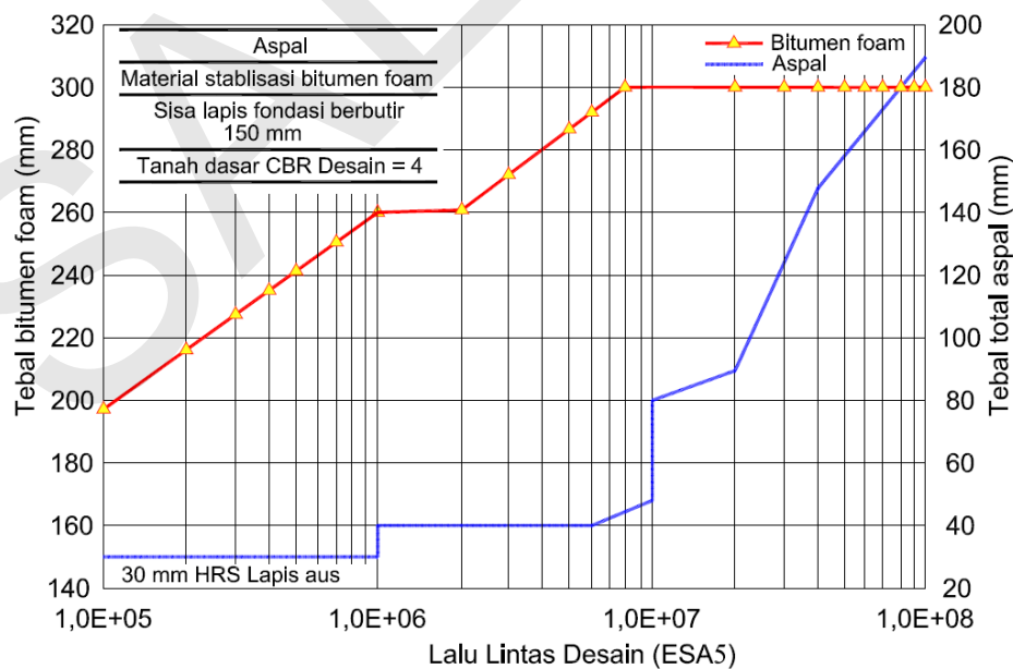
Gambar 8.3. Contoh Bagan Desain Untuk Merancang Tebal Daur Ulang dengan Stabilisasi Foam Bitumen
