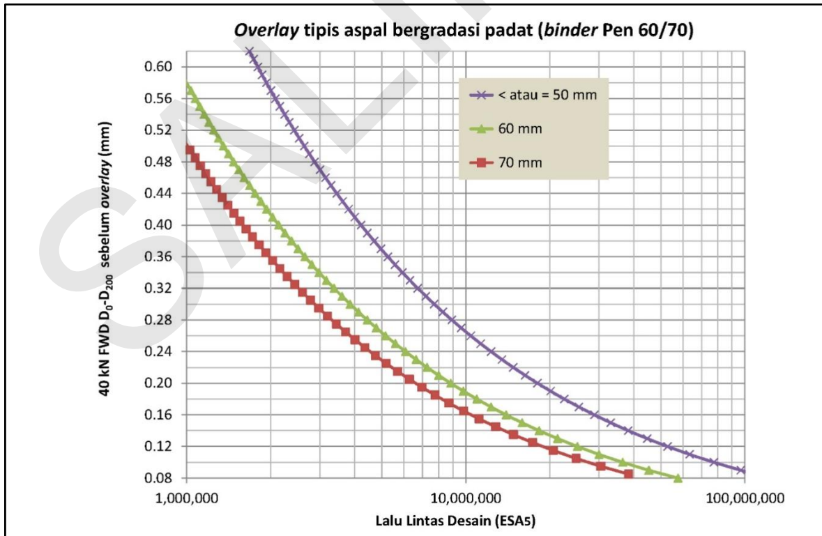
Gambar L.2a. Tebal Overlay Tipis Berdasarkan Lengkung Lendutan (FWD) (Kurva Beban > 20x10 6 ESA5 Hanya Berlaku Untuk Perencanaan Program)
