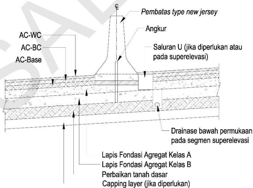
Gambar 8.2. Dukungan Median Perkerasan.
