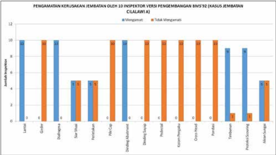
Gambar 3.8 Pengamatan kerusakan jembatan oleh CIA pada elemen level 3
