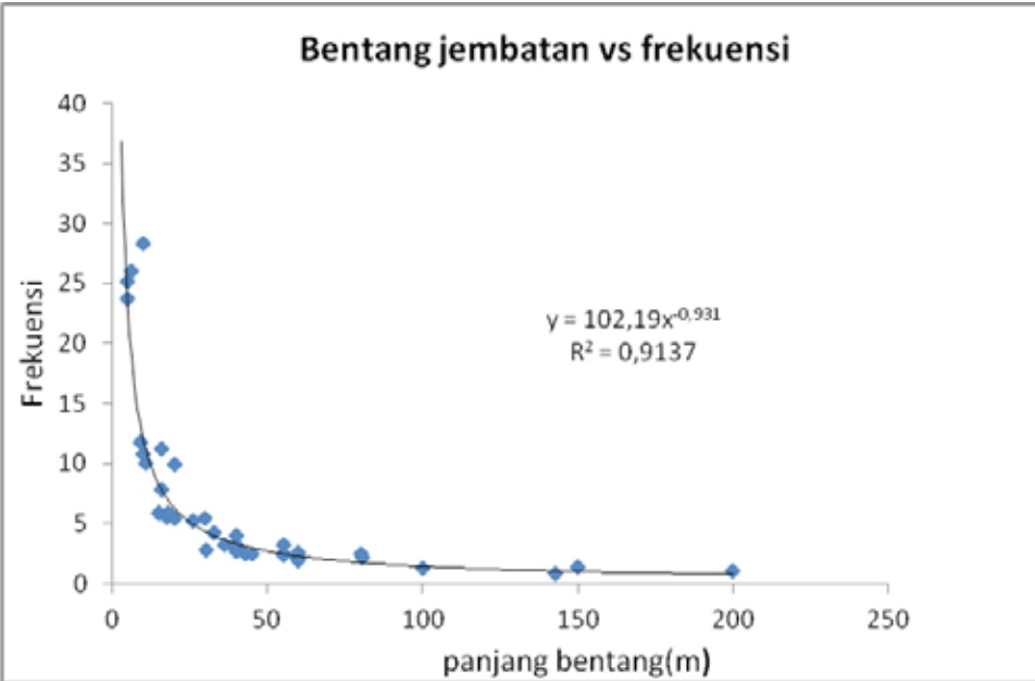
Gambar 4.2 Grafis dari formula empiris frekuensi alami berdasarkan panjang jembatan
