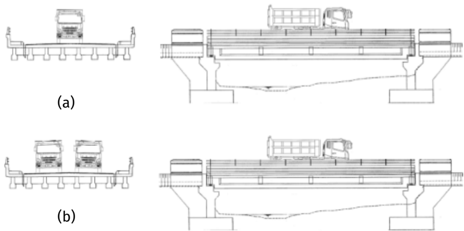
Gambar 4.13 Skema pembebanan
