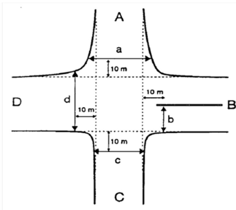
Gambar 2 - Pengidentifikasi masing-masing lengan simpang untuk penentuan jumlah lajur
