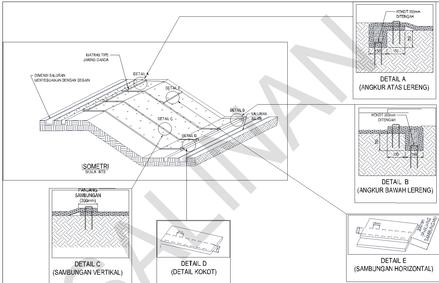
Gambar SKh-3.3.17.5) Ilustrasi Tumpang Tindih ketika Selimut Pengendali Erosi Lereng atau Matras Perkuatan harus Disambung
