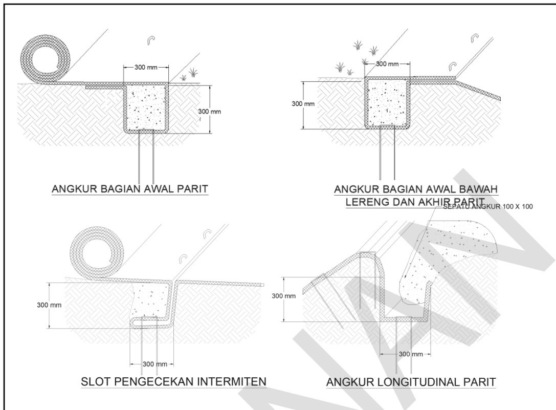
Gambar SKh-3.3.17.4) Ilustrasi Pemasangan Angkur Parit
