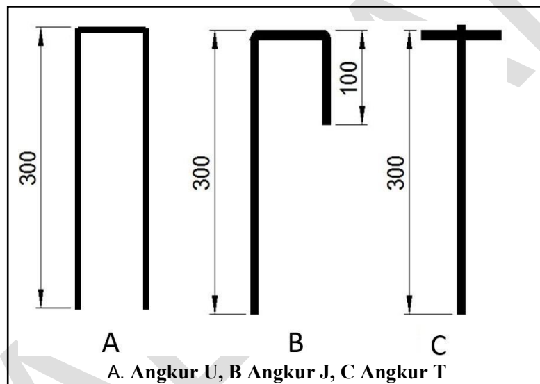
Gambar SKh-3.3.17.3) Ilustrasi Bentuk Angkur (Panjang Terjangkar Minimum 300 mm, Diameter Minimum 8 mm)
